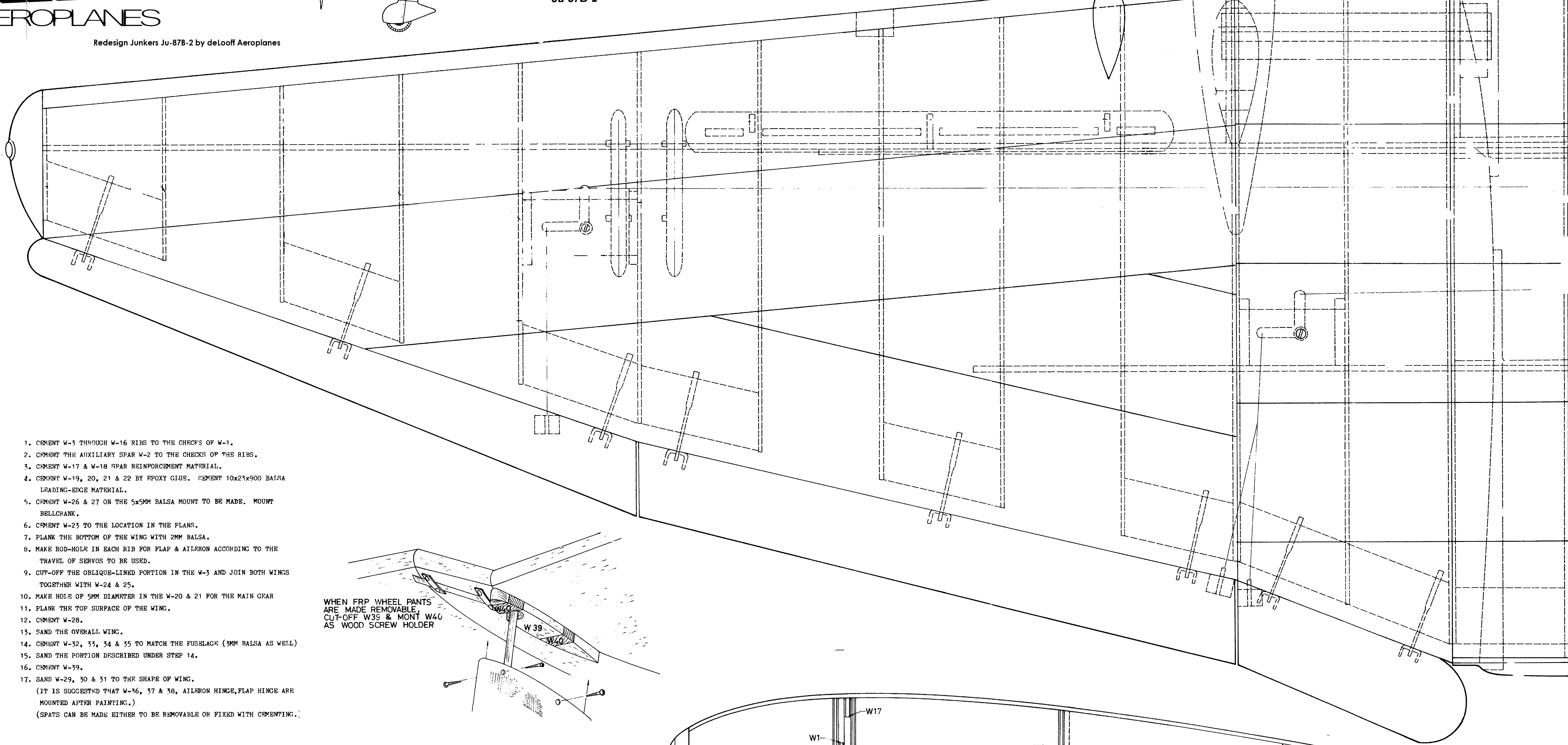
Ju 87B-2
